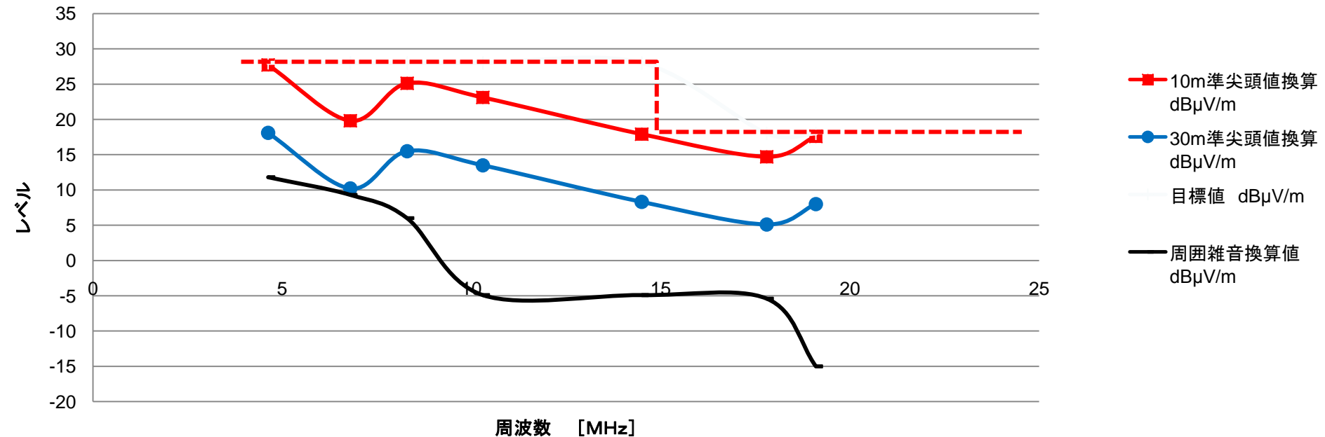
図 ハロックス製PLCモデム漏洩雑音 裾野市 測定点B
