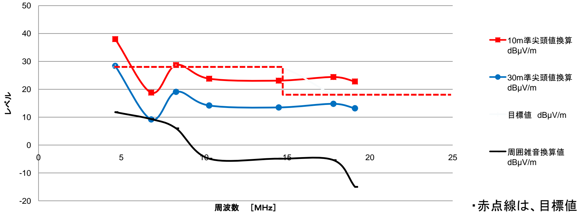
図 ハロックス製PLCモデム漏洩雑音 裾野市 測定点C
