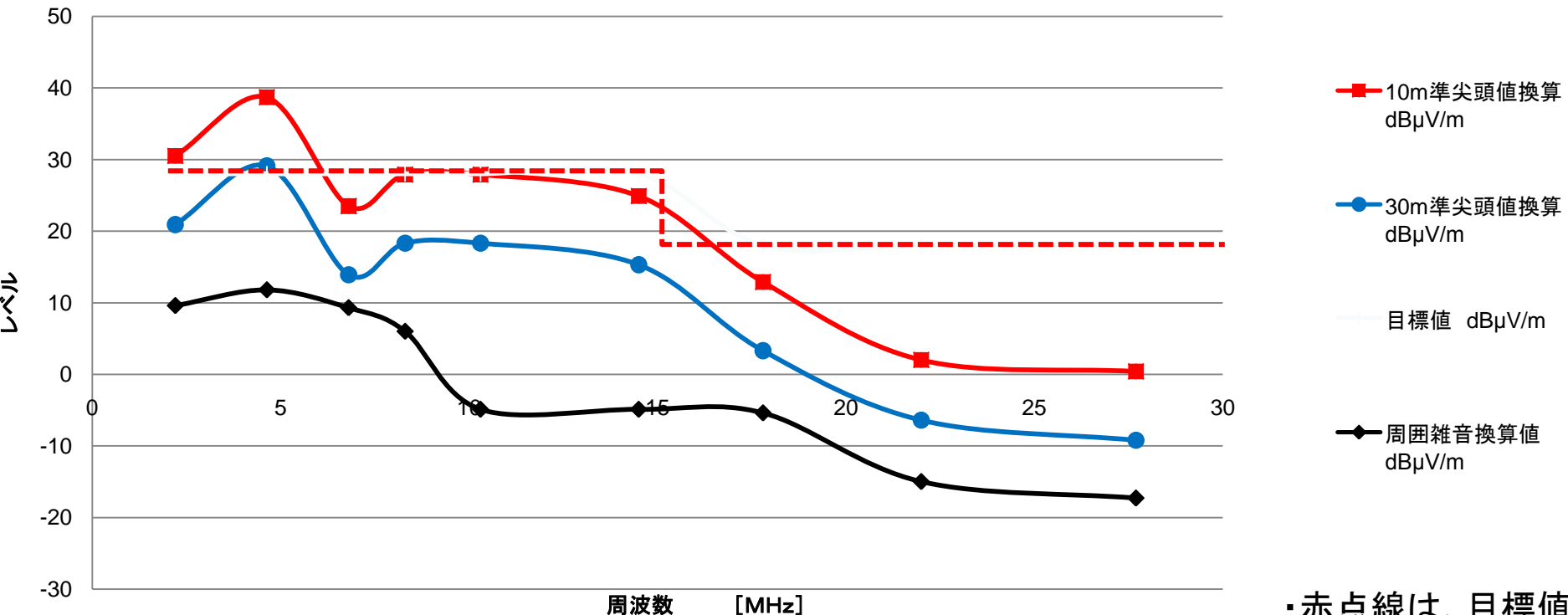
図 パナソニック製PLCモデム漏洩雑音 裾野市 測定点C
