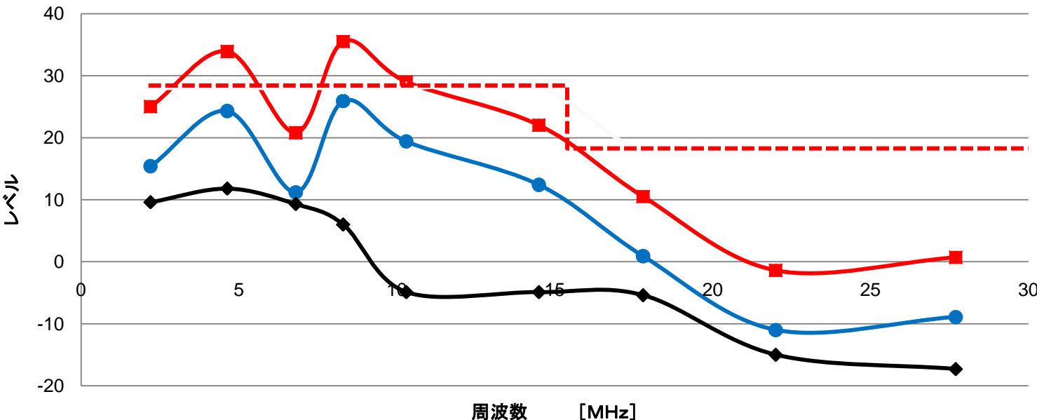
図 パナソニック製PLCモデム漏洩雑音 裾野市 測定点A
