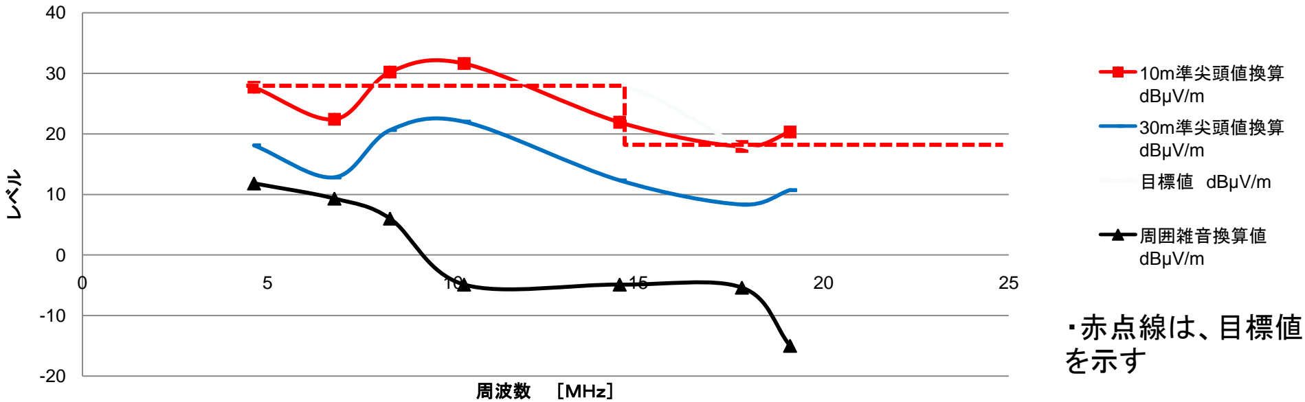
図 ハロックス製PLCモデム漏洩雑音 裾野市 測定点A
