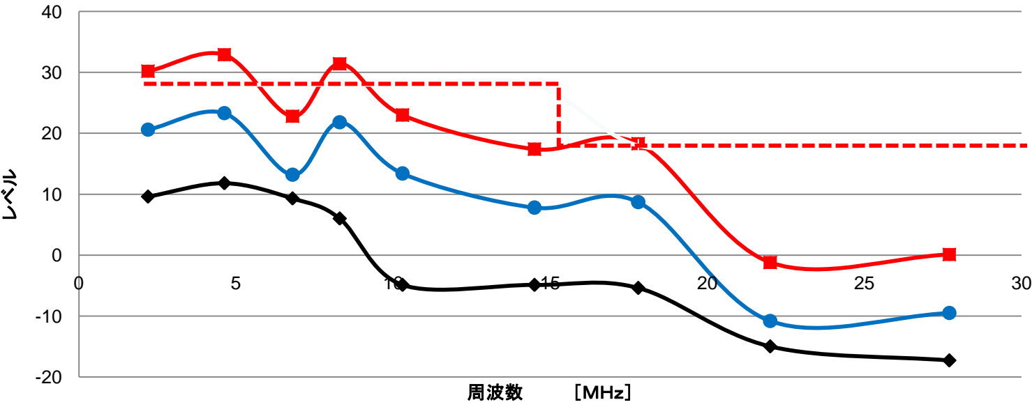
図 パナソニック製PLCモデム漏洩雑音 裾野市 測定点B
